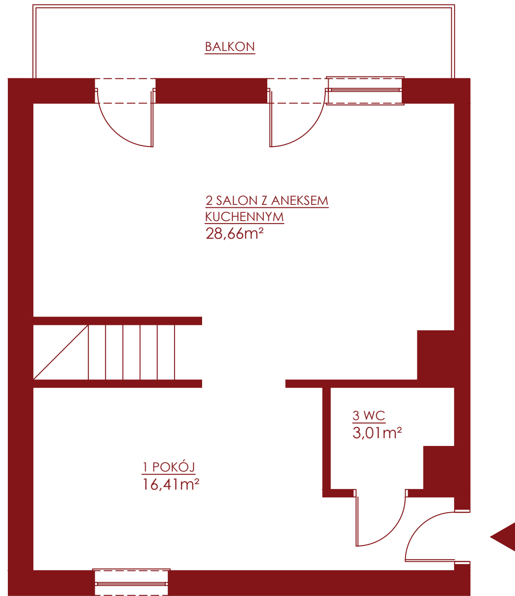
RZUT KONDYGNACJI 5
