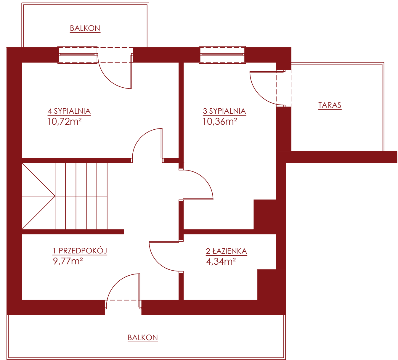
RZUT KONDYGNACJI 6
